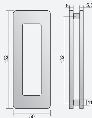
Puxador SGK 02 aço inox e vidro lapidado 01.72.010
